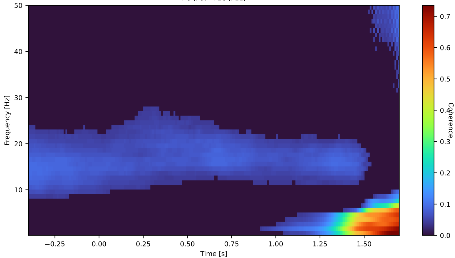
PG (P8) - PEC (P11)
